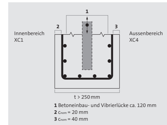
Fig. 28 Détermination de l'épaisseur minimale d'un mur en fonction de l'enrobage, du ferrailage, et du mode de mise en place du béton.
